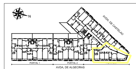
PLANTA PRIMERA PORTAL 3 VIVIENDA B SUPERFICIE UTIL = 94.40 m2
